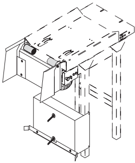
PS Tablettübergabe- Einheit
