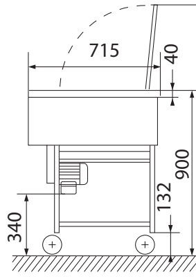
RHIMA Modell 2000 C Seitenansicht (in mm)
