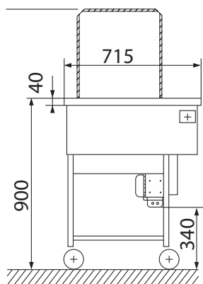
RHIMA Modell 2000 B Vorderansicht (in mm)
