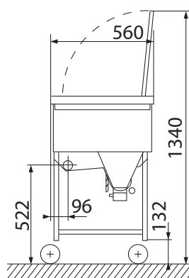
RHIMA Modell 2000 B Seitenansicht (in mm)
