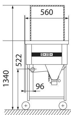
RHIMA Modell 2000 C Vorderansicht (in mm)
